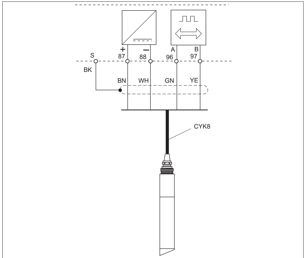
OUS31 和 OUS41 浊度传感器的连接示意图
